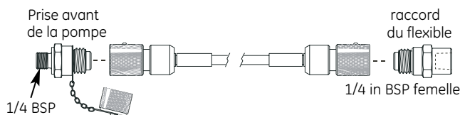
Schéma du HK 15
